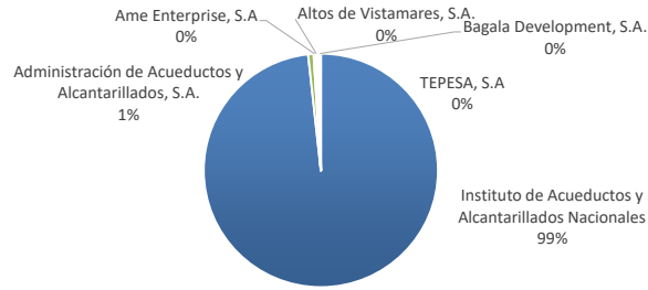
Gráfico 1. PORCENTAJE DE RECLAMOS ADMITIDOS DE AGUA: 2023
